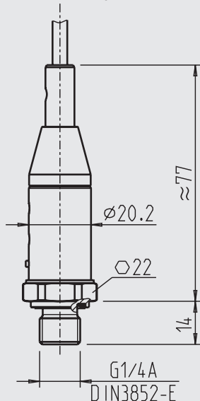
z wyjściem kablowym
